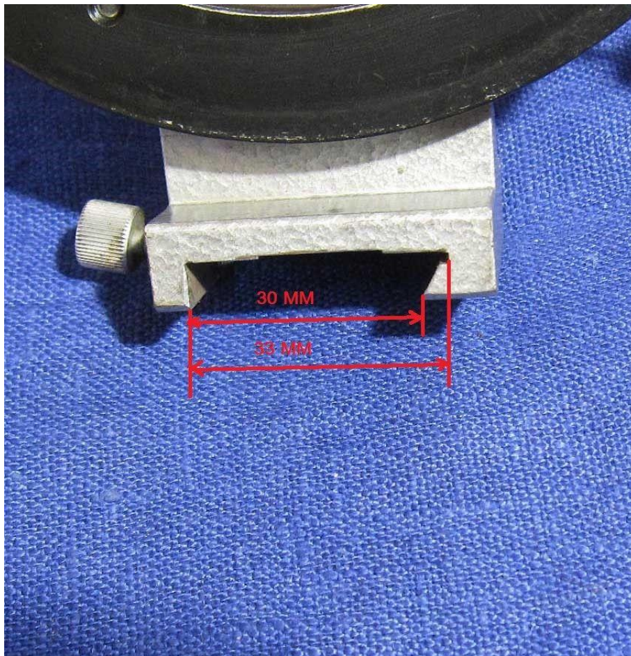
Maße der Befestigungsschwalbe
