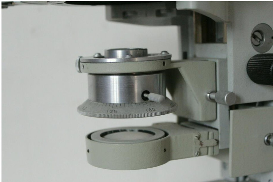
Kondensor mit Polarisator; drehbar mit Skala, sowie Klapplinse. (die obere Abbildung zeigt falsche Montage)
