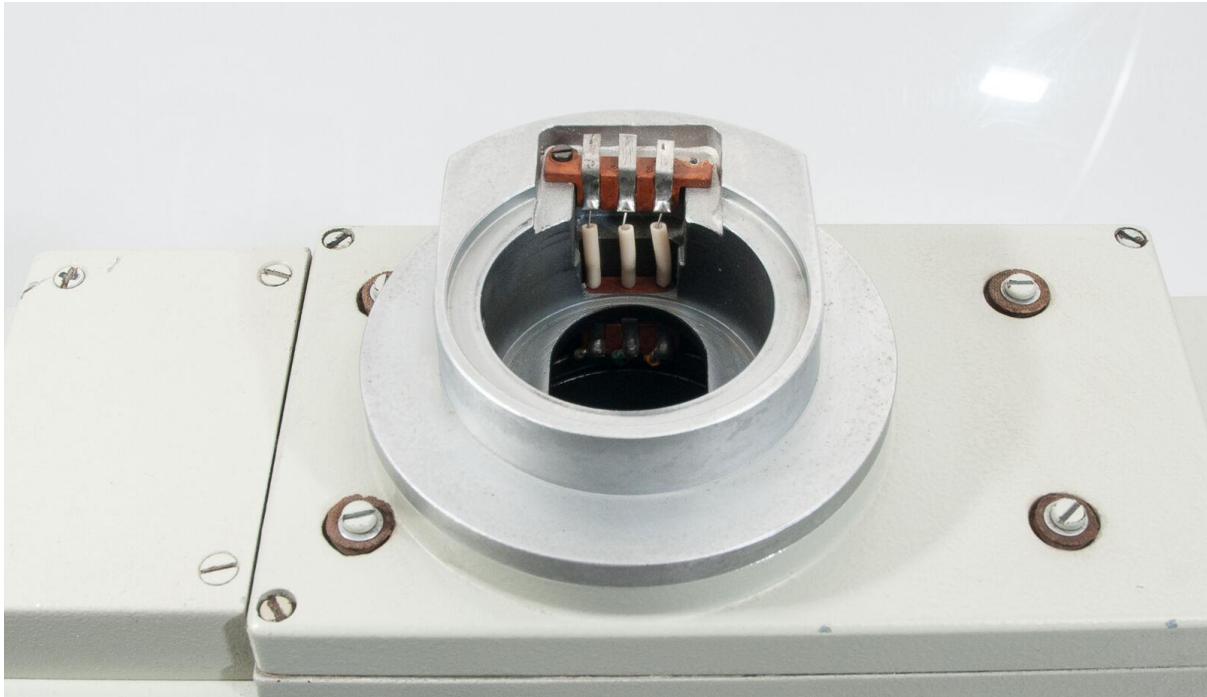
Kameranschluß mit den Kontakten zur Steuerung der Kamera.
