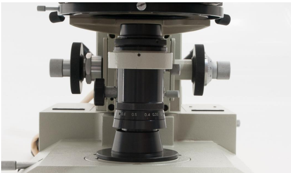
Pankratischer Kondensator PK-3 mit NA 0,2-1,4
