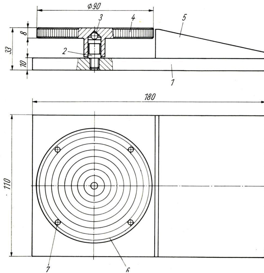
Bild 111. Drehvorrichtung
